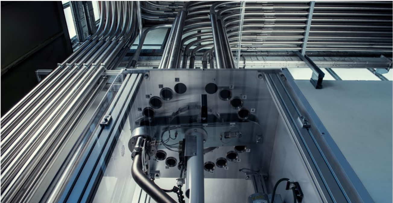
Diramazione del PP alle presse.
